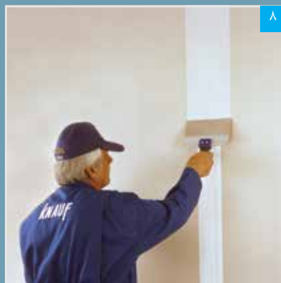
۸ مرحله دوم درزگیری: اجرای لایه دوم بتونه به پهنای ۲۰ سانتیمتر
